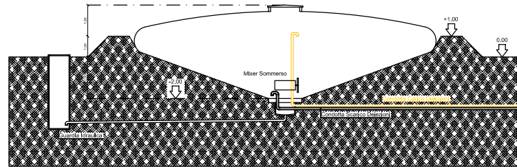
Sezione A:A
